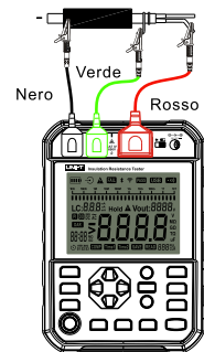
Fig. 10.1.3 Collegamento a tre fili
