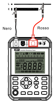
Fig. 9.3.2.1 Collegamento a filo della misura di tensione
