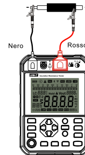
Fig. 10.1.1 Collegamento a due fili
