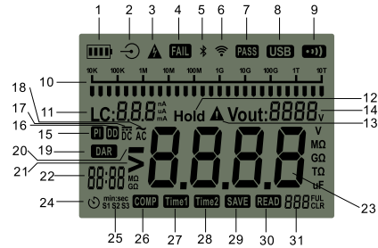
Fig. 7.1 Simboli sul display LCD
